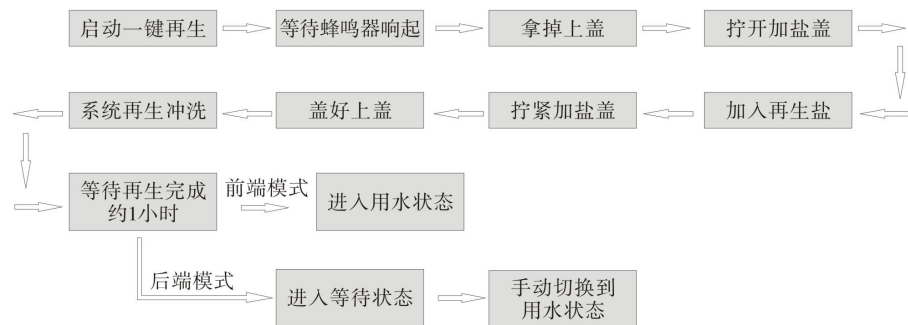
再生过程操作流程图
